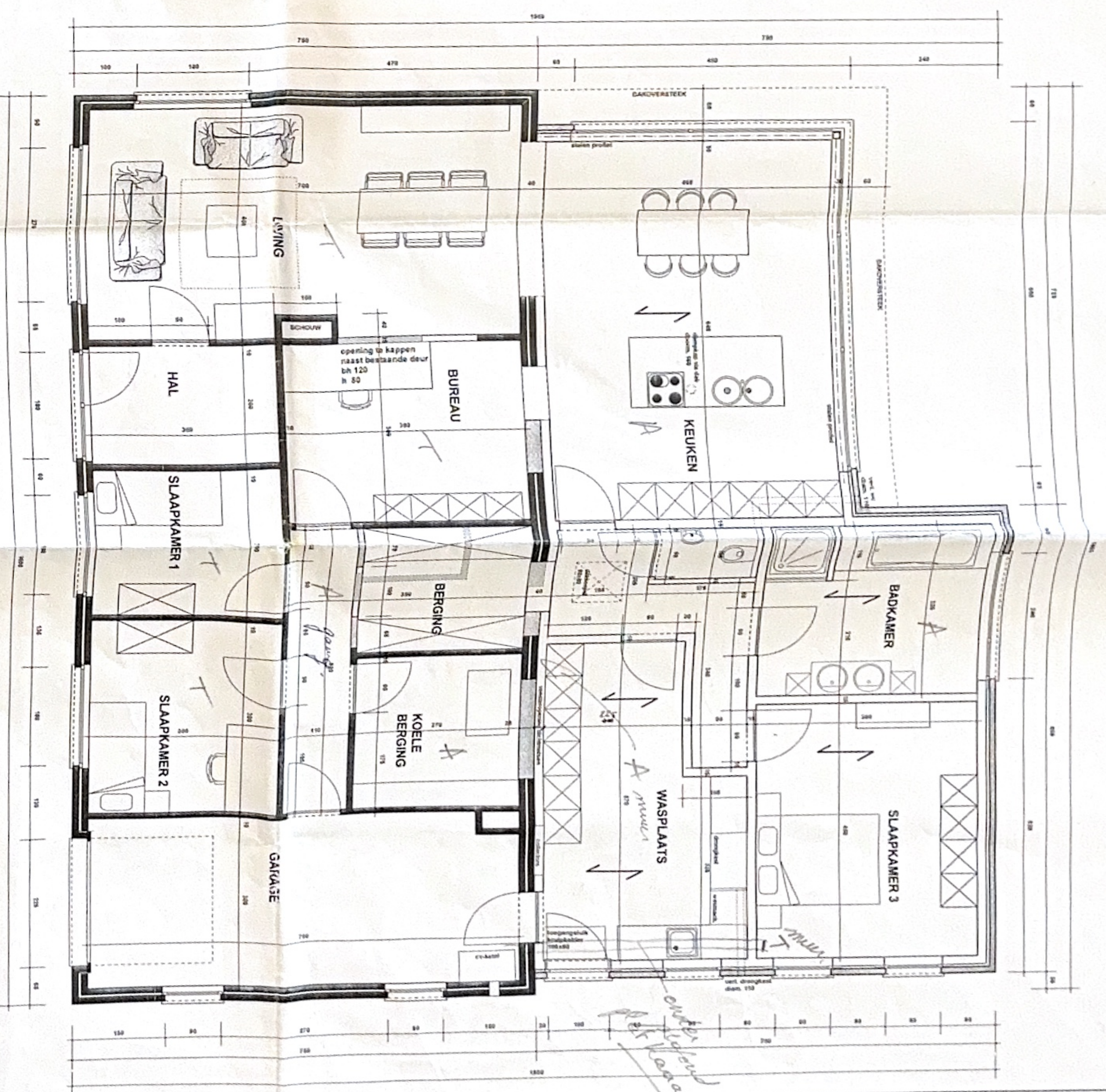
GRONDPLAN schaal 1/50
