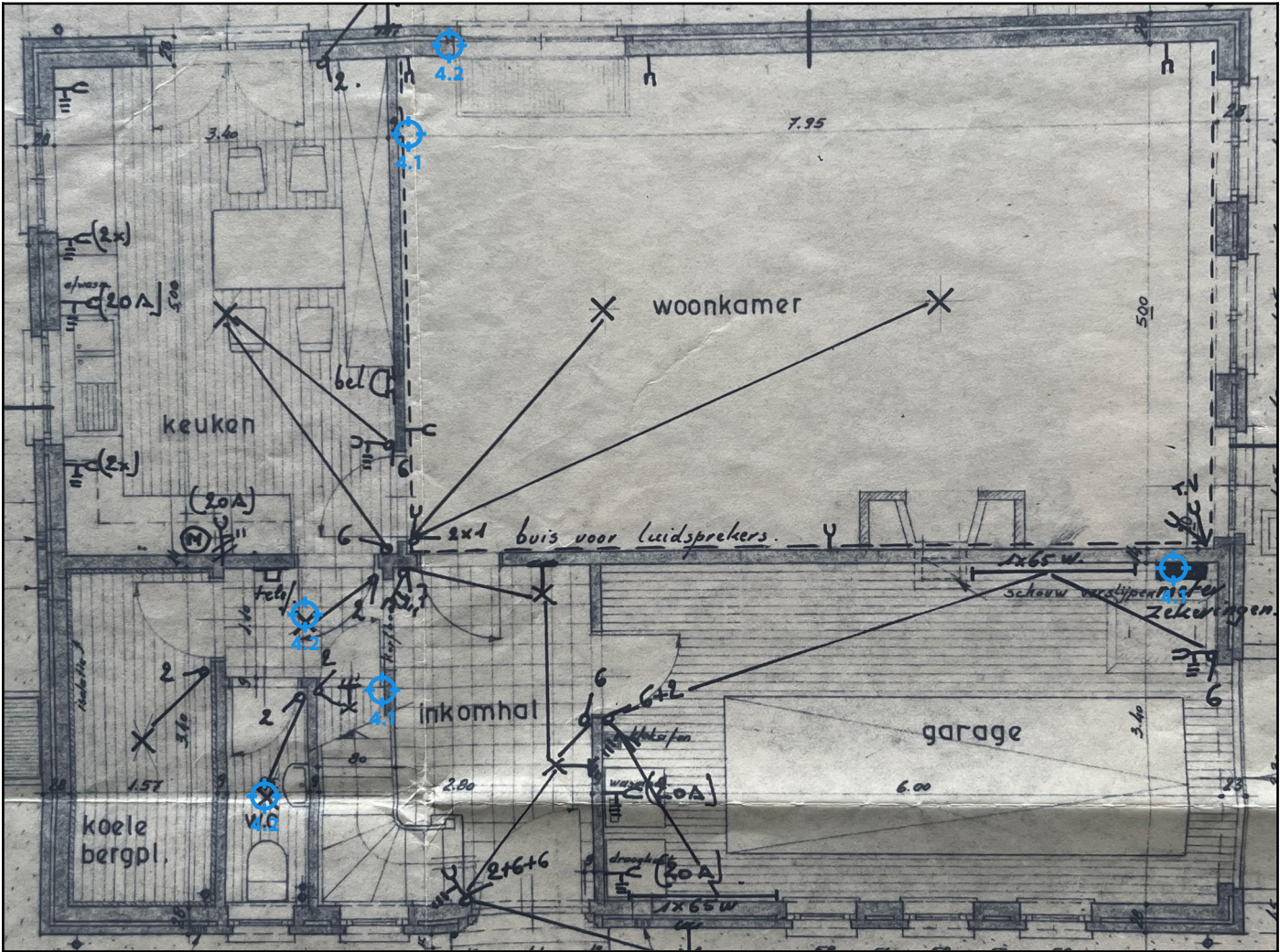
Legende van plan 1.3: Grondplan Gelijkvloers
