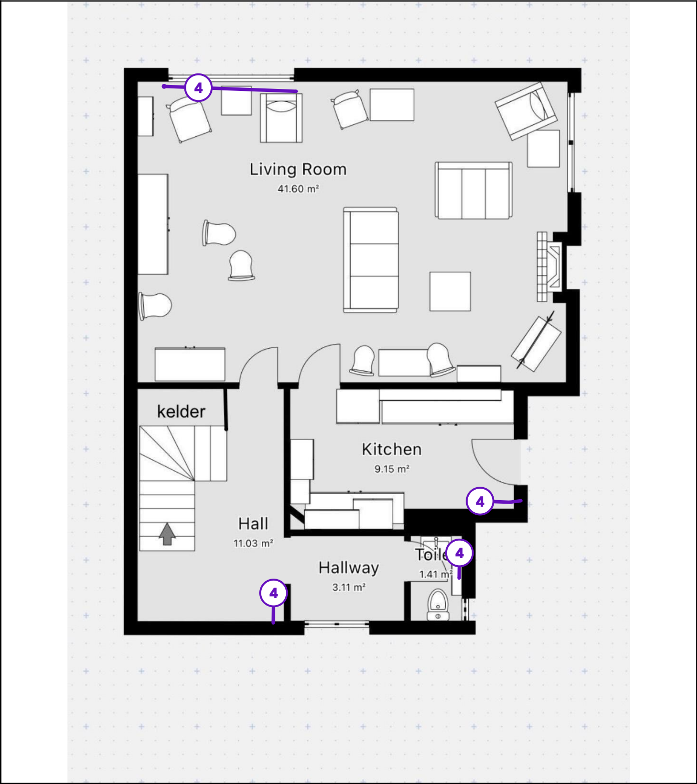
Legende van plan 1.7: Glv grondplan
